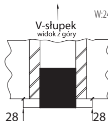
V-słupek W:2458 S:86 G:68
