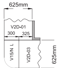
Przykładowe zastosowanie regału narożnego V-15/N
